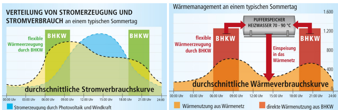
Abb. 37: Prinzip netzdienliche Fahrweise BHKW
