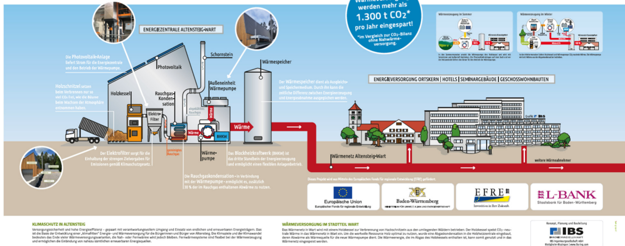
Abb. 34: Beispiel Heizzentrale Altensteig-Wart mit Hackschnitzelheizung und Wärmepumpe (Wärmepumpe: Sommer Außenluft / Winter Abgaskondensation)
