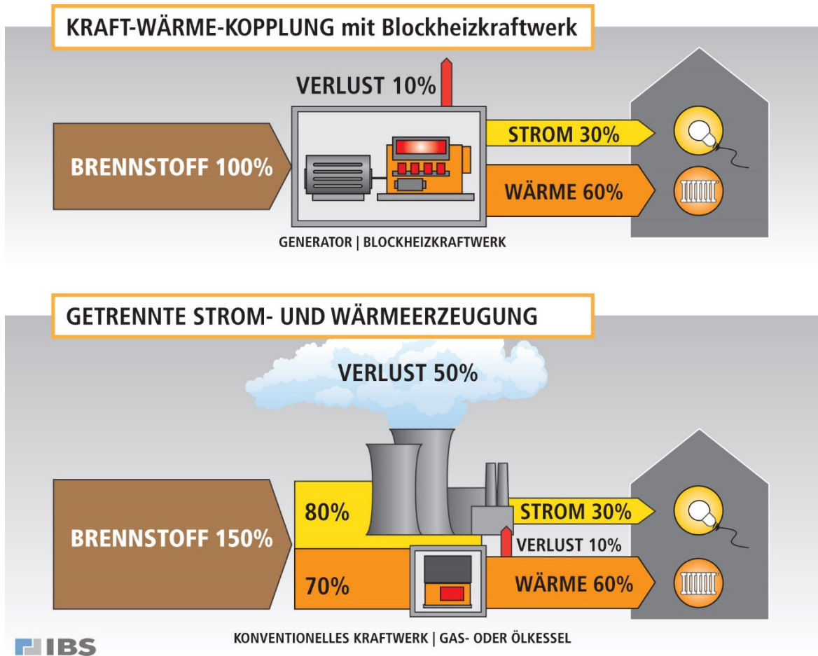
Abb. 36: Prinzip Kraft-Wärme-Kopplung im Vergleich zu getrennter Strom- und Wärmeerzeugung
