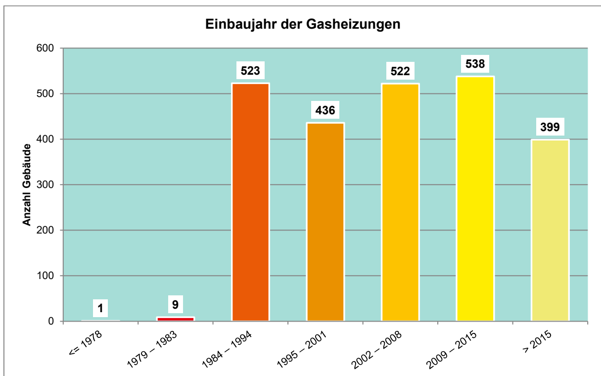
Abb. 18: Verteilung der erfassten Erdgas-Einzelheizungsanlagen nach Einbaujahr
