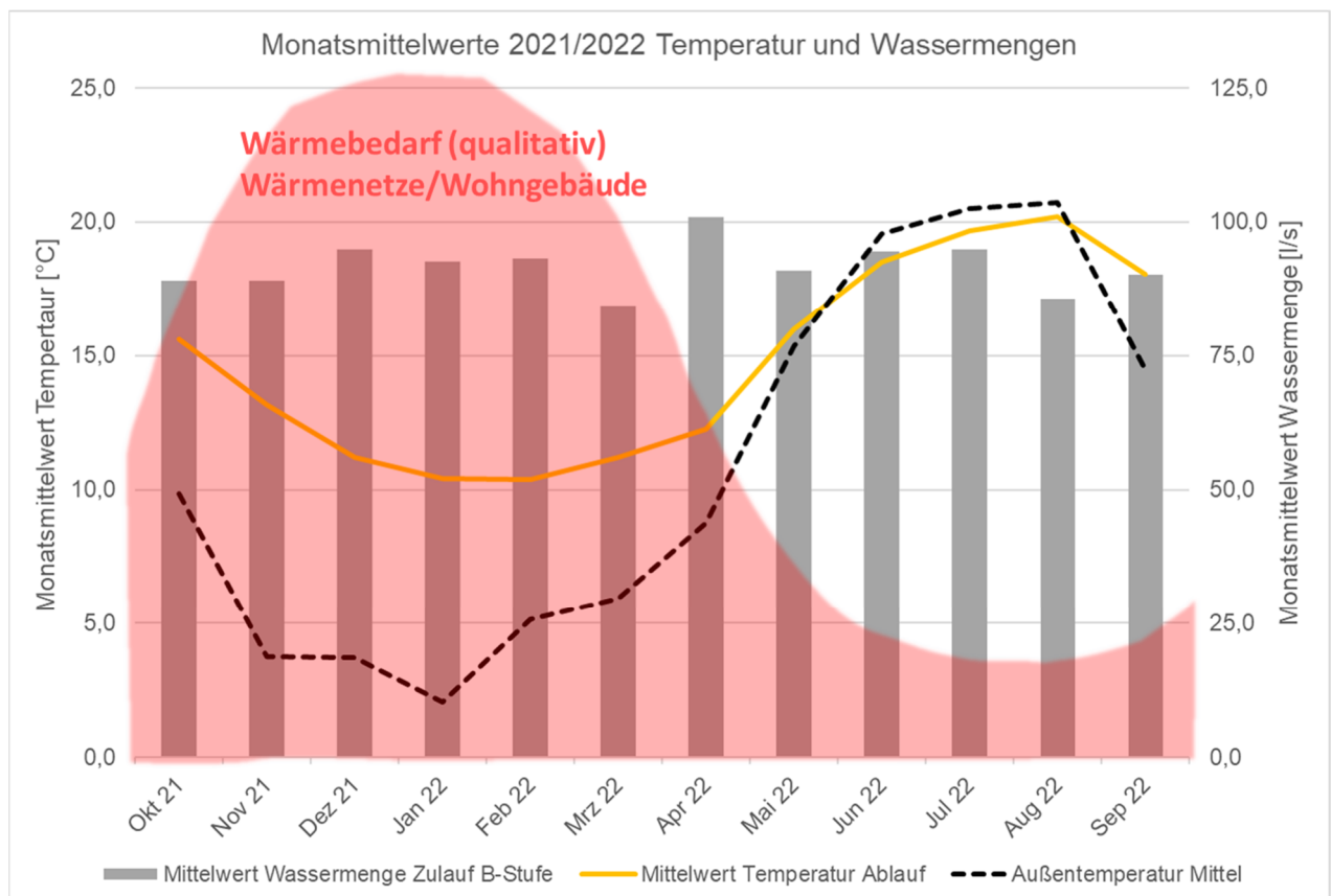
Abb. 40: Volumenstrom Zulauf B-Stufe und Abwasser- sowie Außenlufttemperatur im Monatsmittel Kläranlage Kiebingen 2021/22
