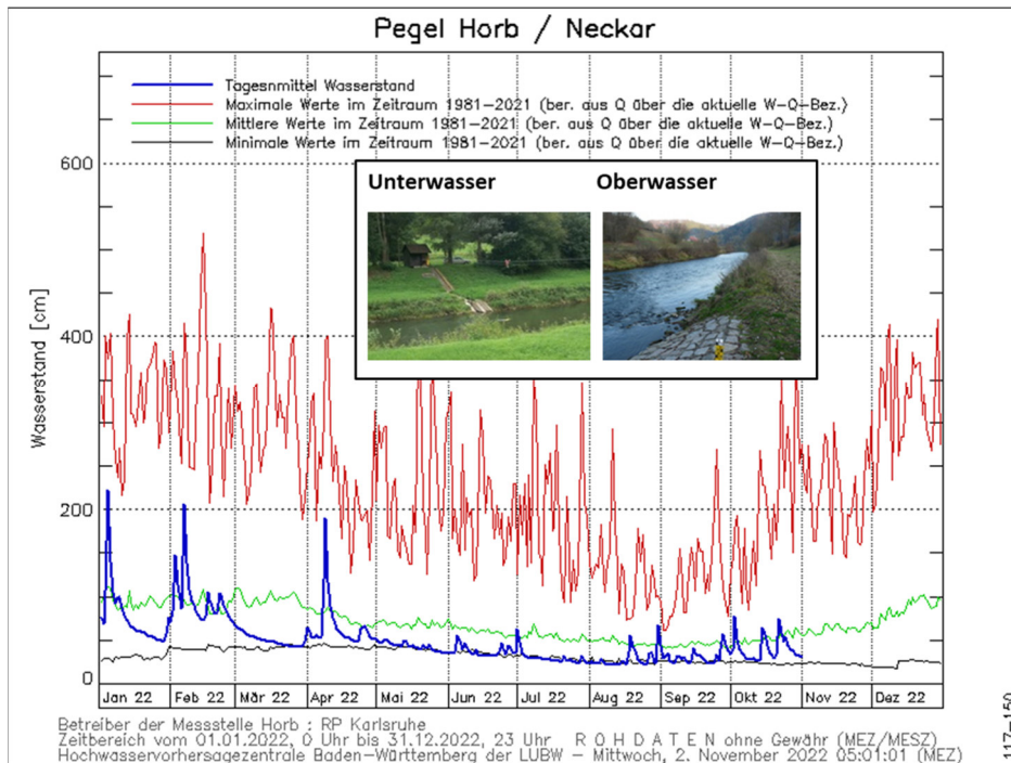
Abb. 44: Wasserstandsmessungen am Neckar (Messstelle Horb 2022 und historisch) - Quelle: www.hvz.baden-wuerttemberg.de (LUBW)
