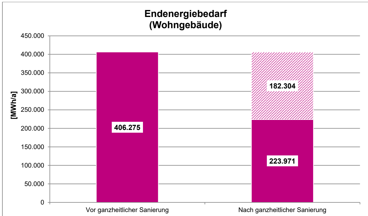
Abb. 23: Einsparpotenzial Endenergiebedarf Wohngebäude (für Wärme) durch bauliche Gebäudemodernisierung
