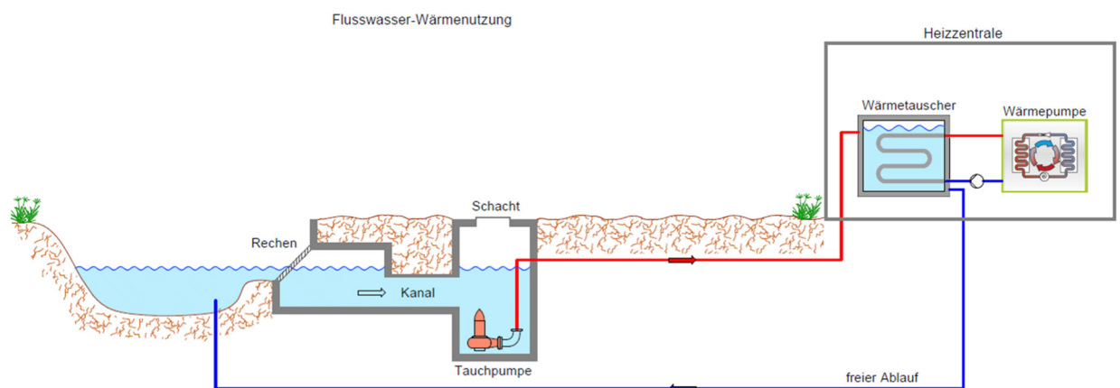
Abb. 46: Prinzipschema Flusswasserwärmepumpe
