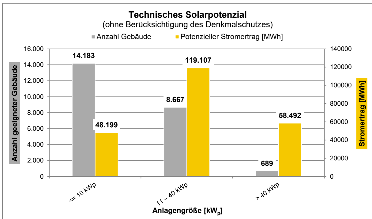
Abb. 52: Anzahl und Stromerzeugungspotenzial möglicher PV-Dachanlagen in Rottenburg nach Anlagengröße
