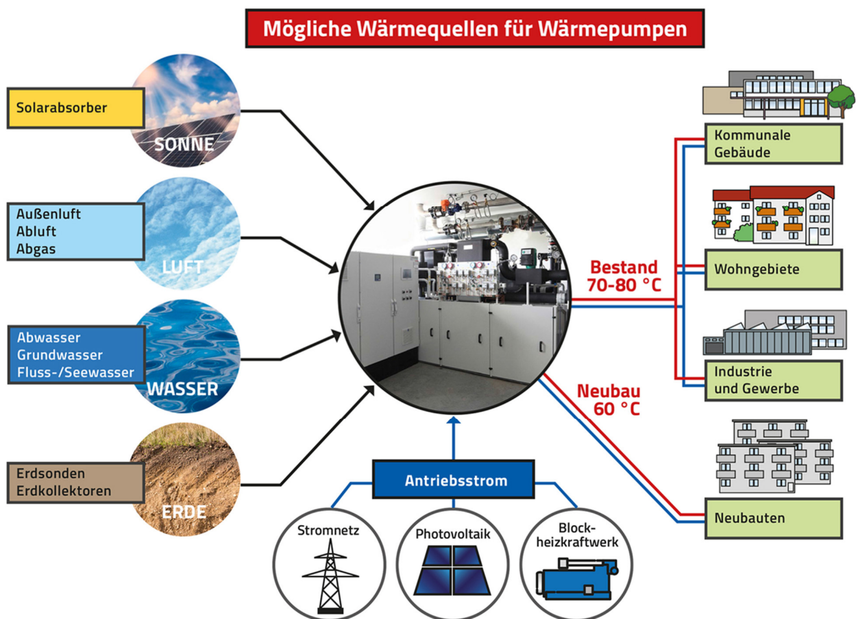
Abb. 38: Wärmequellen für Wärmepumpen
