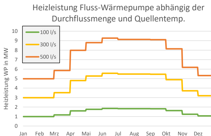
Abb. 41: Mögliche Heizleistungen von Flusswasserwärmepumpen
