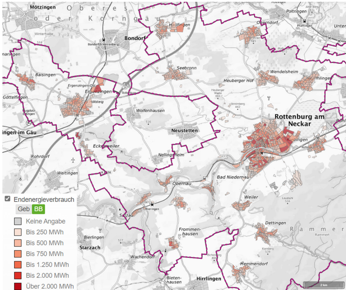
Abb. 7: Endenergiebedarf (Wärmeversorgung) auf Baublockebene
