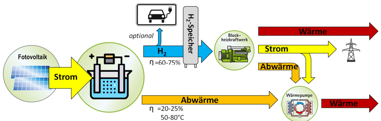
Abb. 48: Prinzipschema saisonale Wasserstoffspeicherung (Auszug Beratungsbericht IBS)
