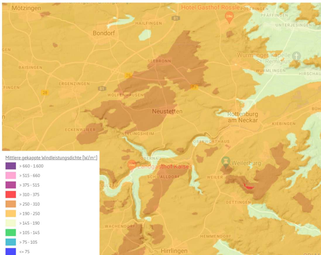
Abb. 59: mittlere gekappte Windleistungsdichte (Darstellungen: www.energieatlas-bw.de)
