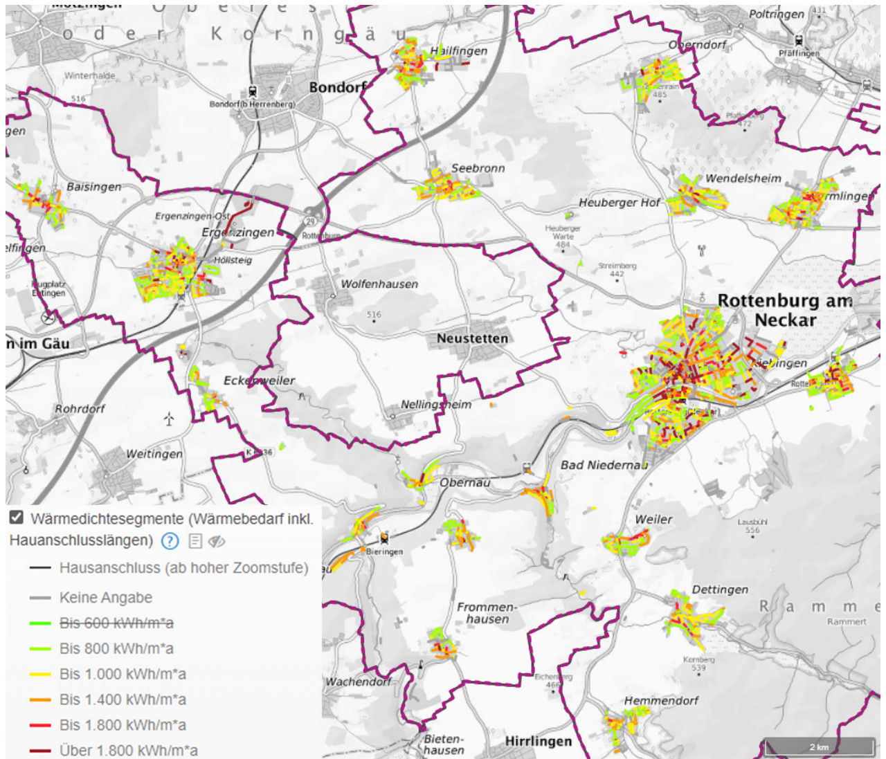
Abb. 9: Wärmeverbrauchsichte von Straßenabschnitten
