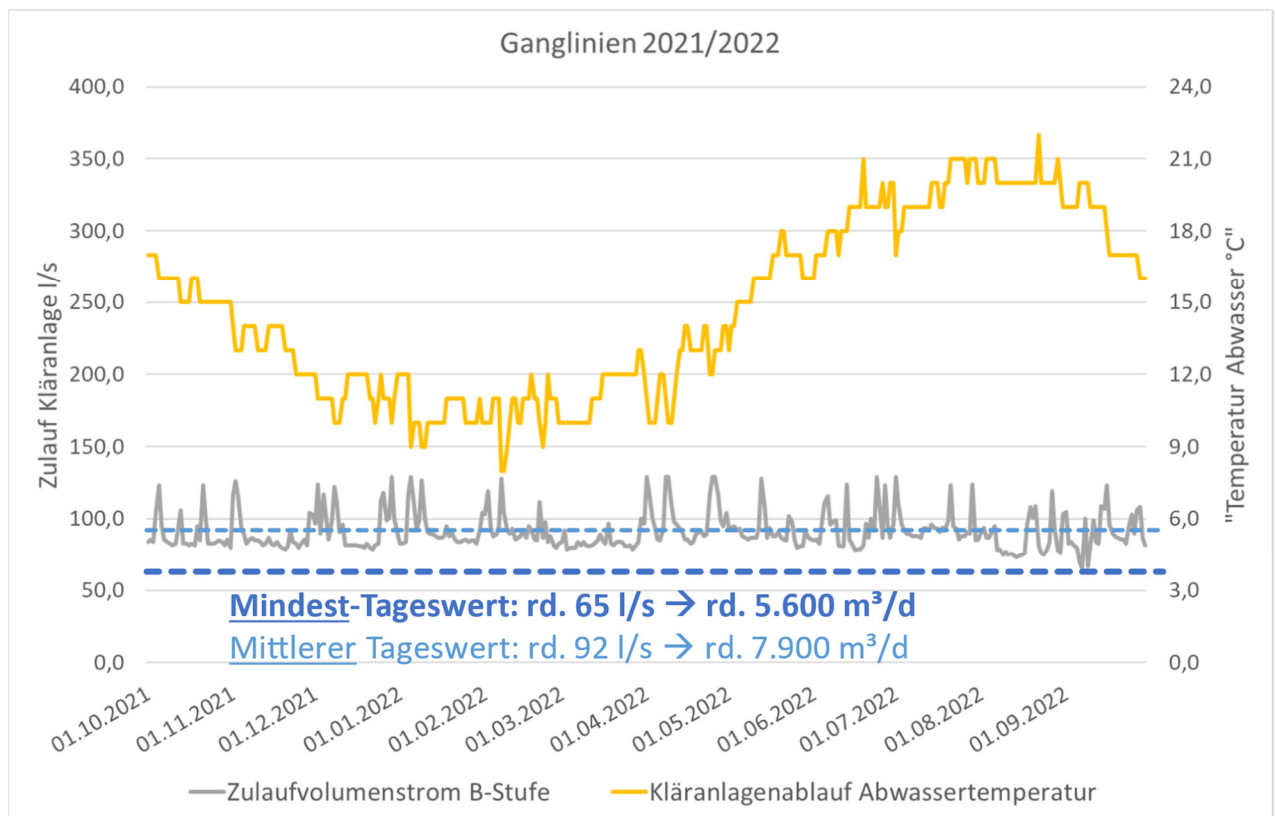
Abb. 39: Zulauf Belebungsstufe und Abwassertemperatur Kläranlage Kiebingen Okt. 2021 – Sept. 2022
