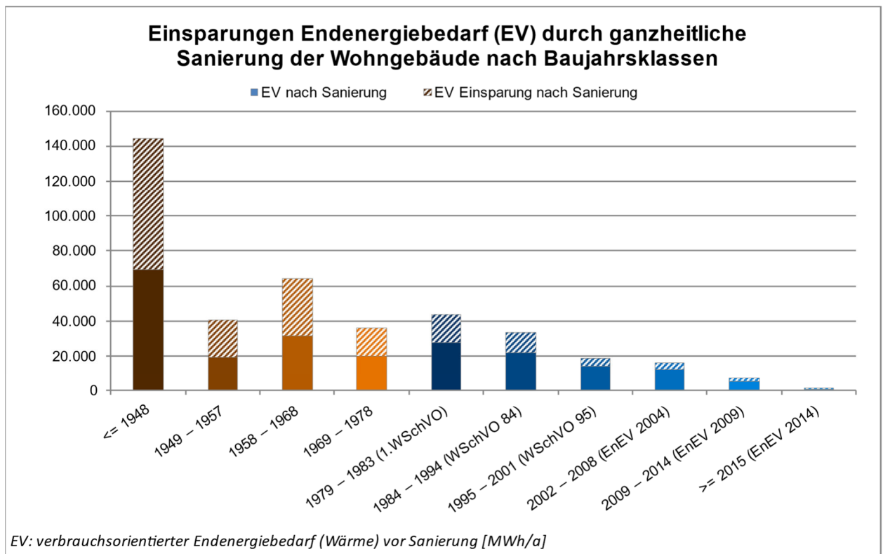
Abb. 25: Einsparpotenziale Endenergie der Wohngebäude nach Baualtersklasse
