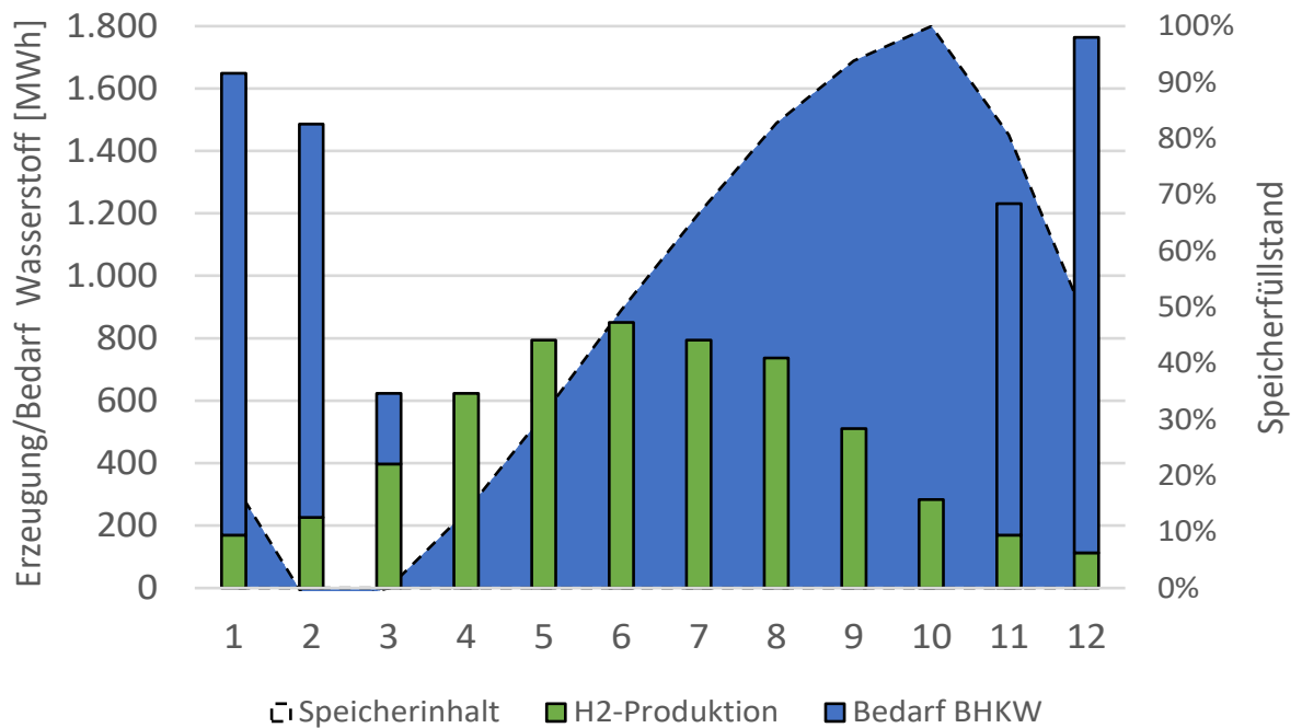
Abb. 51: Wasserstoffbilanz saisonaler H 2 -Speicher (Auszug Beratungsbericht IBS)
