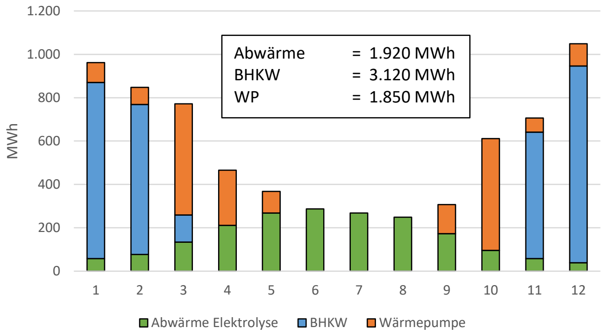
Abb. 50: Beispiel monatliche Wärmebilanz saisonaler H 2 -Speicher mit H 2 -BHKW (Auszug Beratungsbericht IBS)
