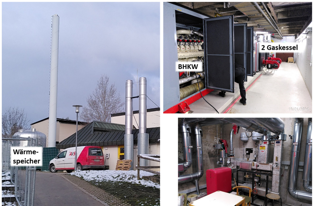
Abb. 12: Heizzentrale Hohenbergschule
